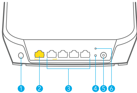
Routeur Orbi
