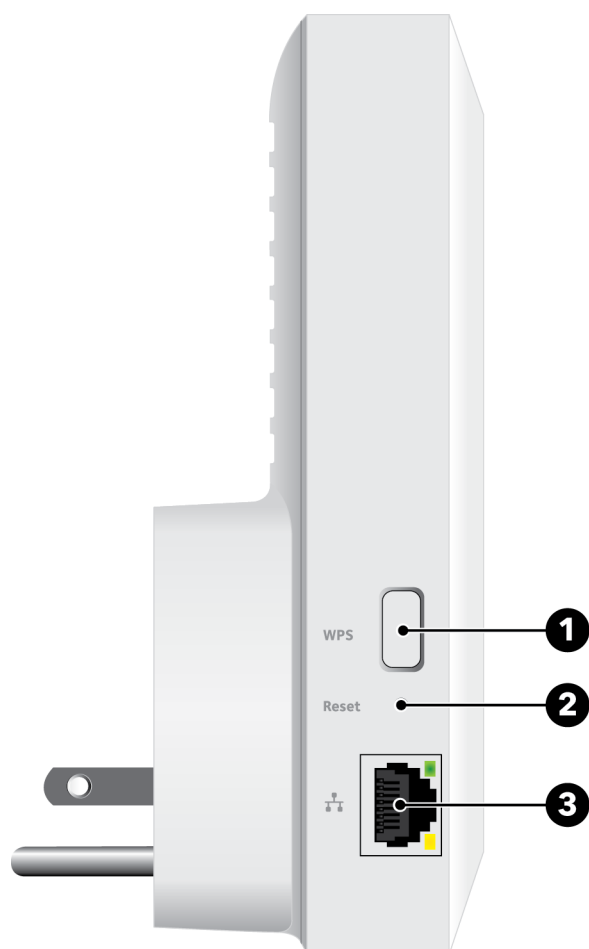
Illustration 3 : Panneau arrière.
