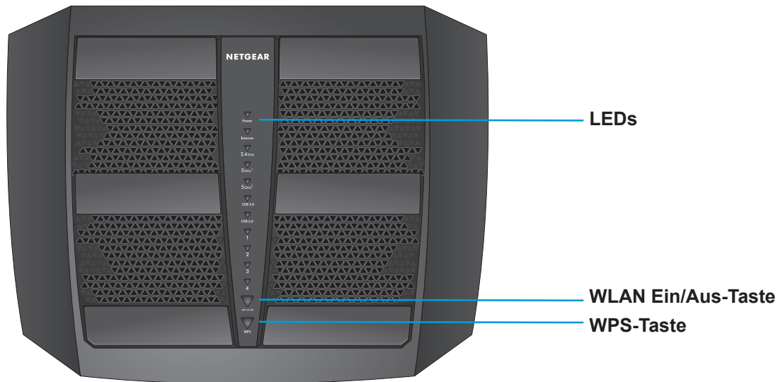
Abbildung 2. Router-LEDs und Tasten
