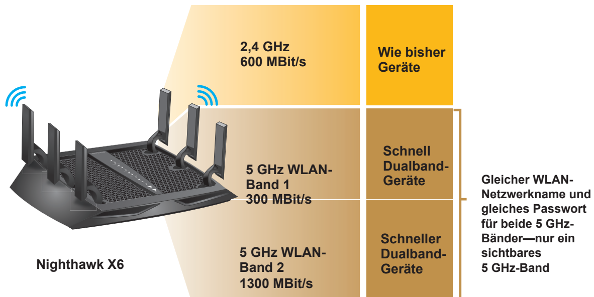
Abbildung 11. Smart Connect
