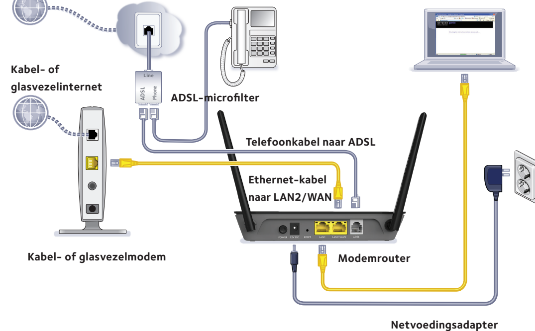
DSL-internet
